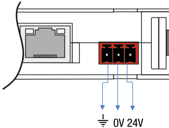
Şekil 4.8 - 24 VDC konektörü
