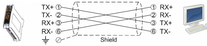
Şekil 13.3 - PC çapraz kablo bağlantısı
