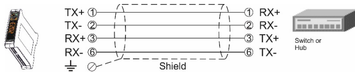
Şekil 16.2 - HUB bağlantısı
