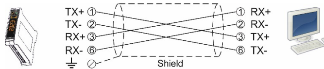
Şekil 14.3 - Çapraz kablo bağlantısı
