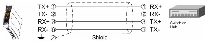
Şekil 13.2 - HUB bağlantısı
