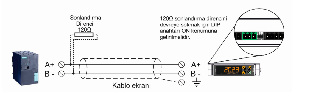
Şekil 4.4 - RS 485 seri arayüz bağlantısı
